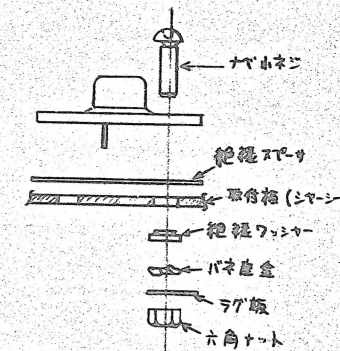
I.C の取付方法
