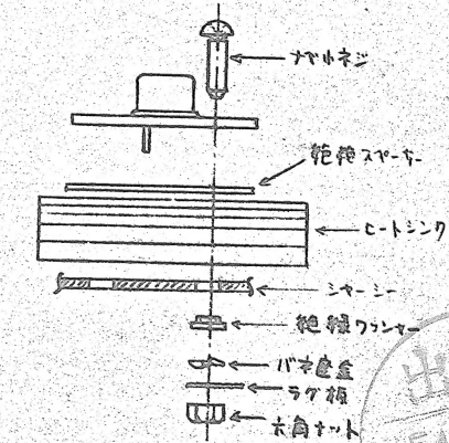
TRの取付方法
