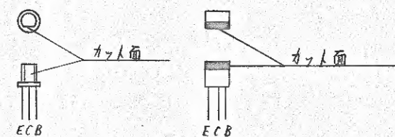
注 コンデンサー取付方法
