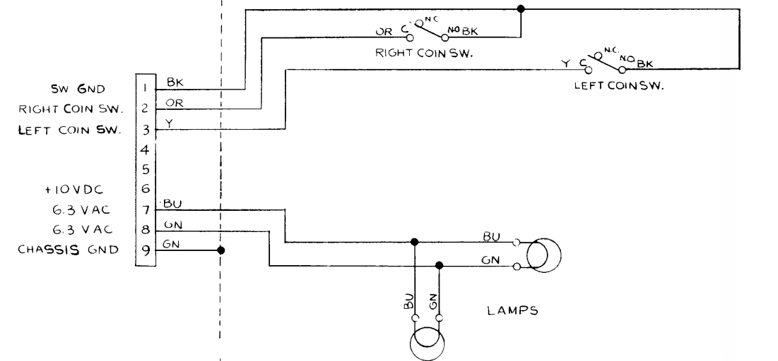
Coin Door Wiring Diagram
